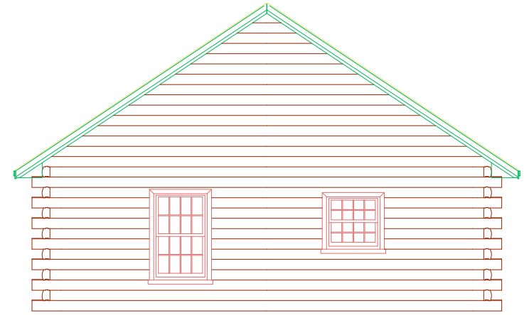
Right Elevation
